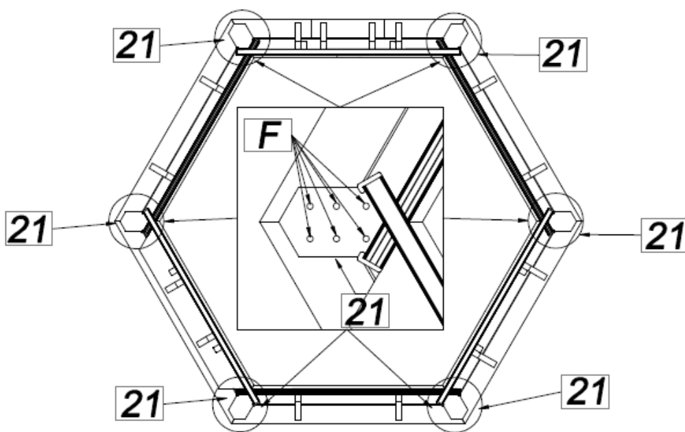
Vista inferior de las cofias
